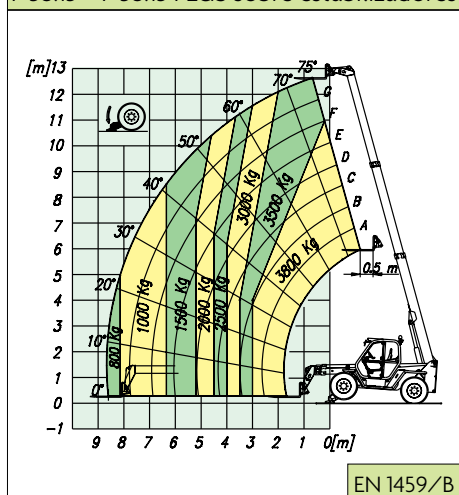
P 38.13 + P 38.13 PLUS sobre estabilizadores
