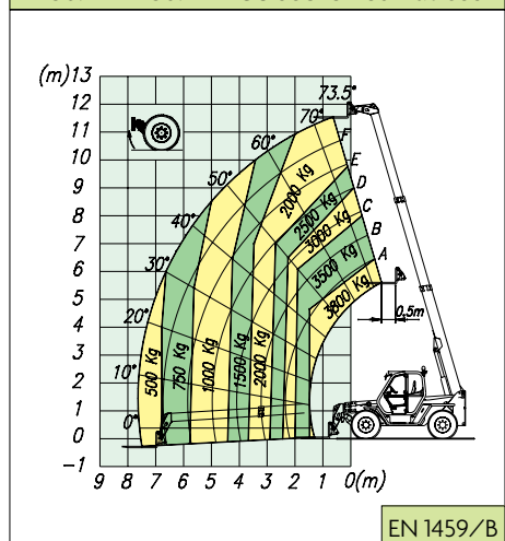
P 38.12 + P 38.12 PLUS sobre neumáticos
