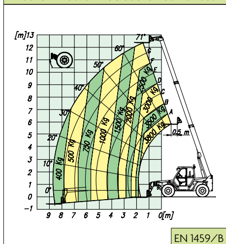
P 38.13 + P 38.13 PLUS sobre neumáticos
