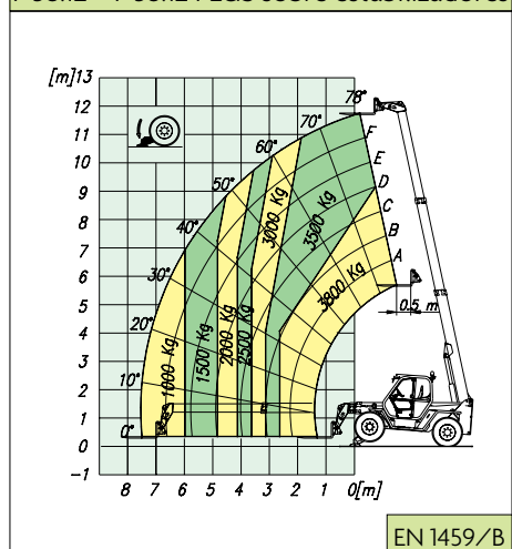
P 38.12 + P 38.12 PLUS sobre estabilizadores
