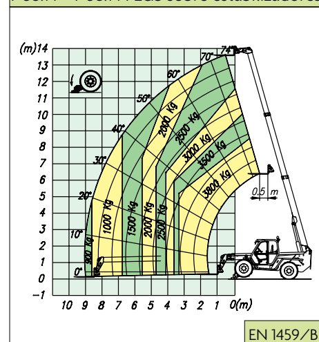
P 38.14 + P 38.14 PLUS sobre estabilizadores
