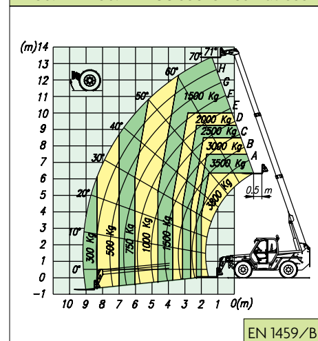
P 38.14 + P 38.14 PLUS sobre neumáticos
